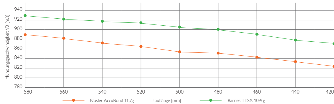
Mündungsgeschwindigkeit in Abhängigkeit zur Lauflänge
